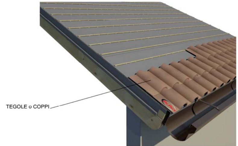
10) ANCORAGGIO TEGOLE o COPPI
