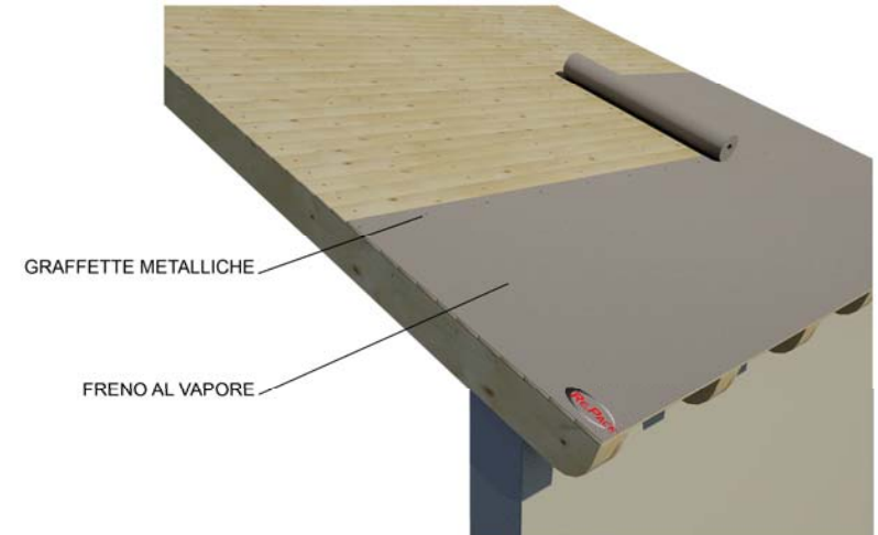
2) STESURA FRENO AL VAPORE
