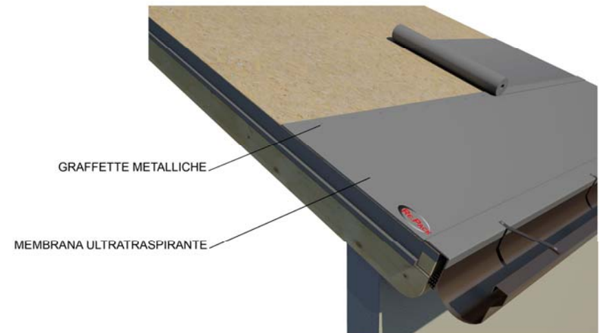
8) STESURA MEMBRANA ULTRATRASPIRANTE
