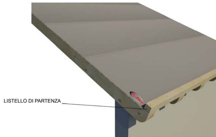
3) INSTALLAZIONE LISTELLO DI PARTENZA
