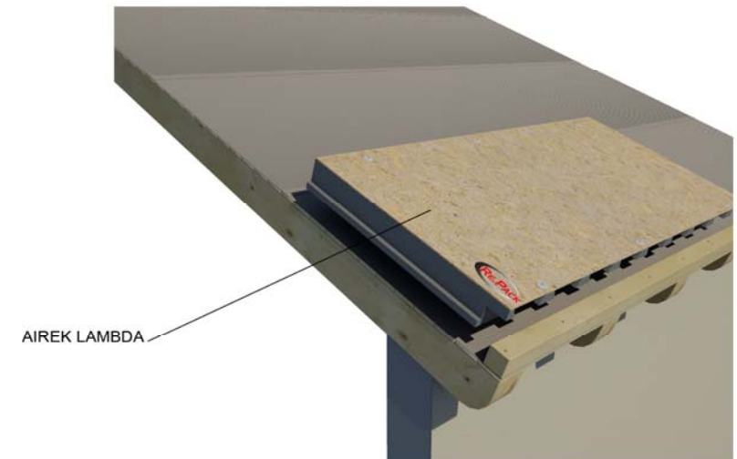
4) INSTALLAZIONE PANNELLO DI PARTENZA GRONDAIA
