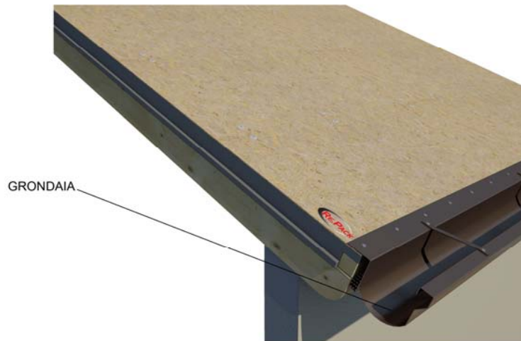
7) INSTALLAZIONE GRONDAIA
