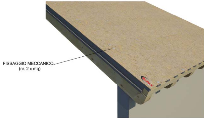
5) FISSAGGIO AIREK LAMBDA
